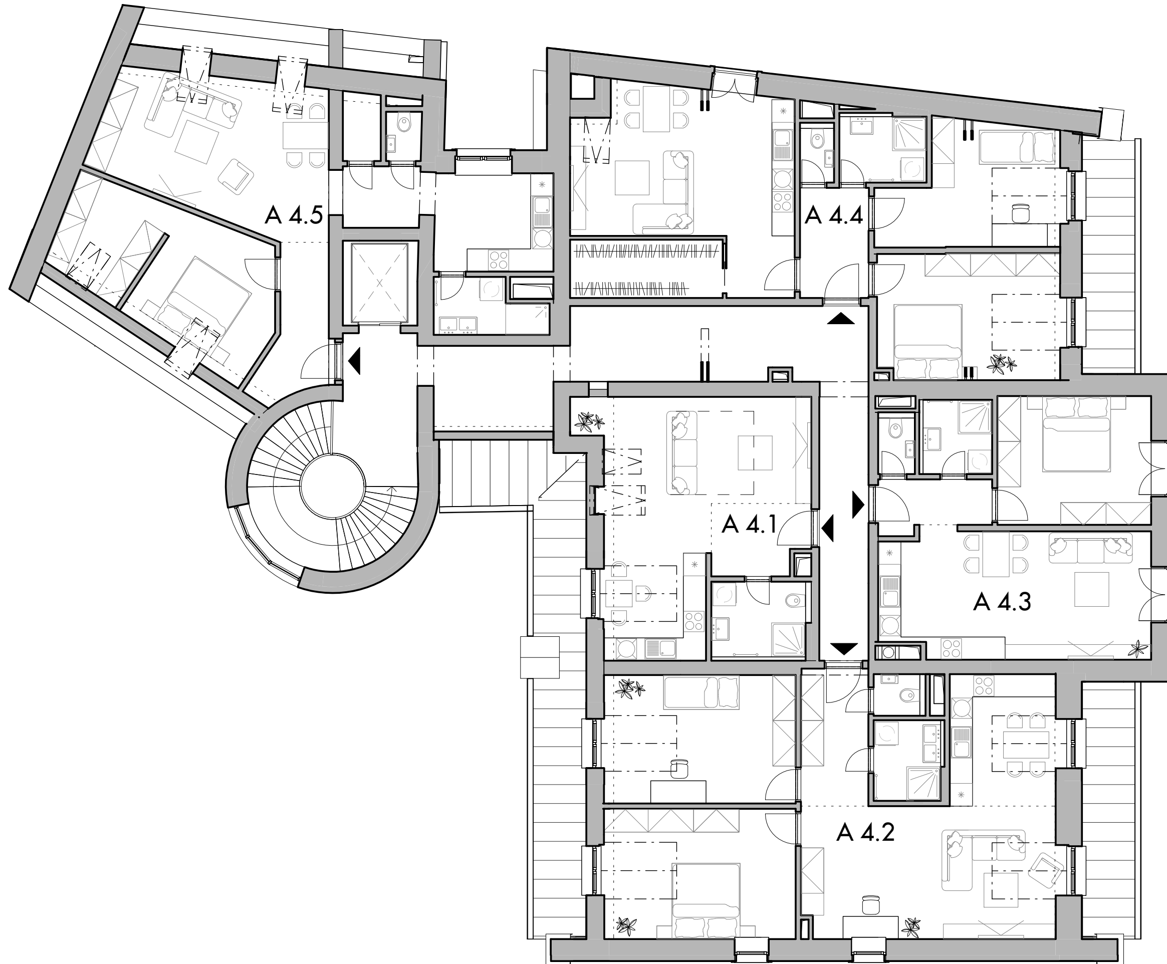
PÔDORYS 4NP- A
